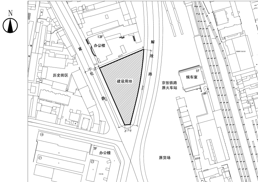
地形图 1:1000
